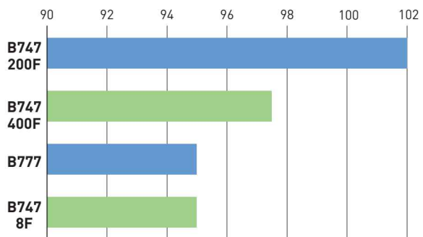
ノイズレベルの機材別比較
