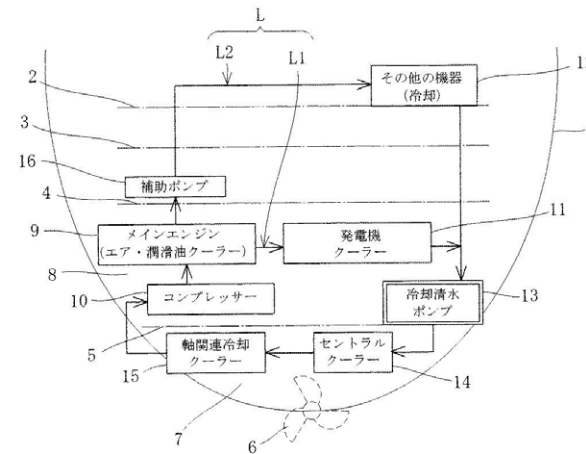
■ 清水系冷却システムの模式図
