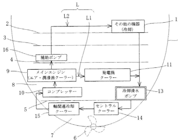
■ 清水系冷却システムの模式図
