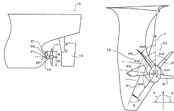
■ 船用推進効率改善装置を備えた船舶の概略構成
