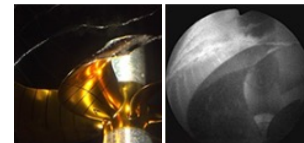
模型プロペラの水槽試験
